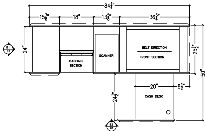
P1 01 PLAN VIEW: SB-208 CHECKOUT LEFT HAND SHOWN SCALE: 3/8" = 1'-0"
